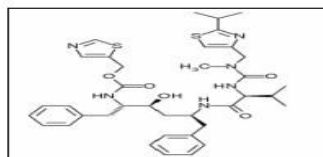
B: Ritonavir
