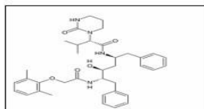
A: Lopinavir
